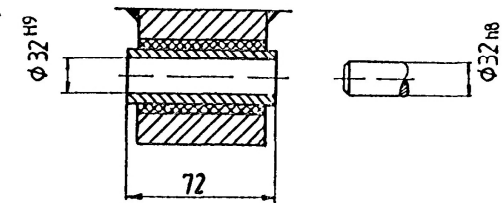
Schnitt C-D
